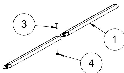
Наращивание трубок.
